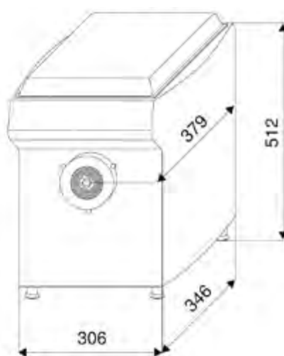
Dimensions Rubis
